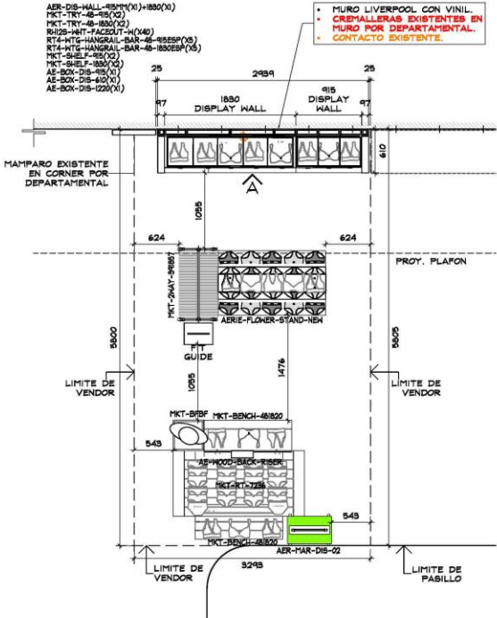
PLANTA ARQUITECTONICA ESC. 1:50
