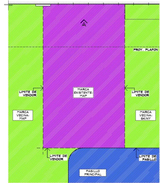
PLANTA GENERAL ESC. 1:50
