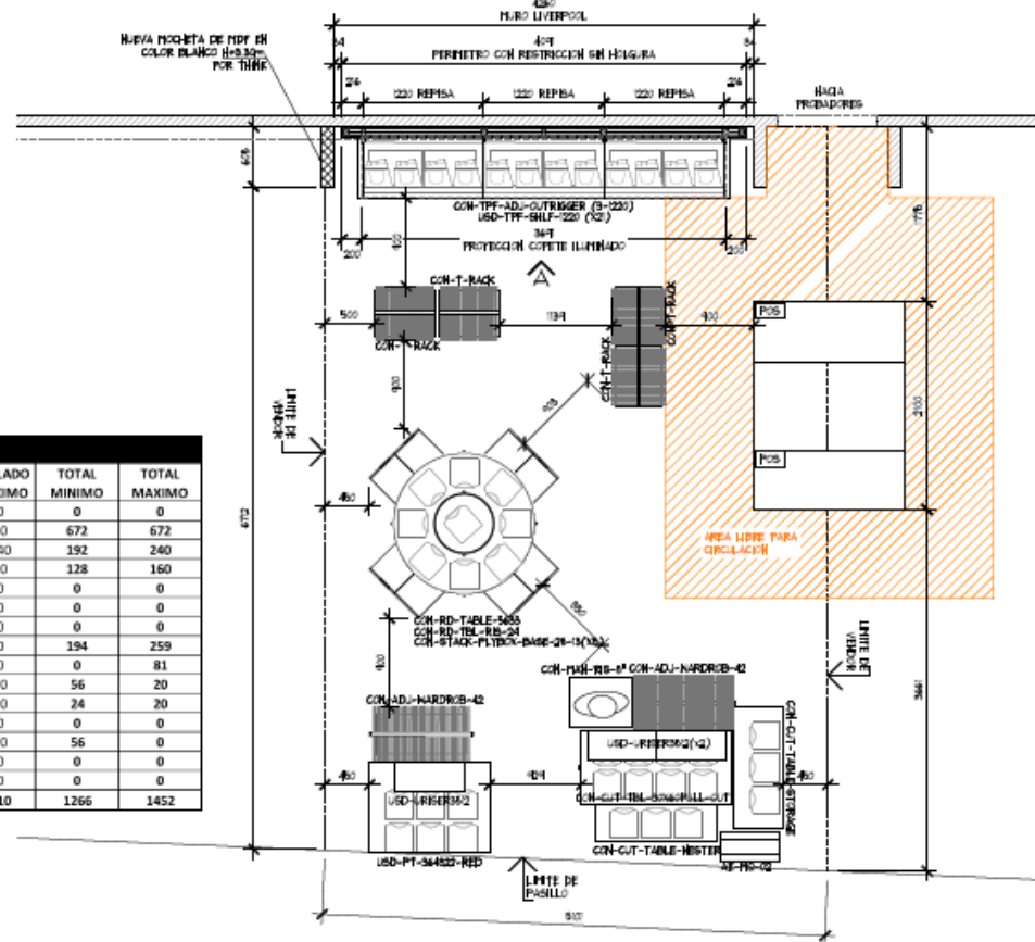
PLANTA ARQUITECTONICA ESC. 1:50
