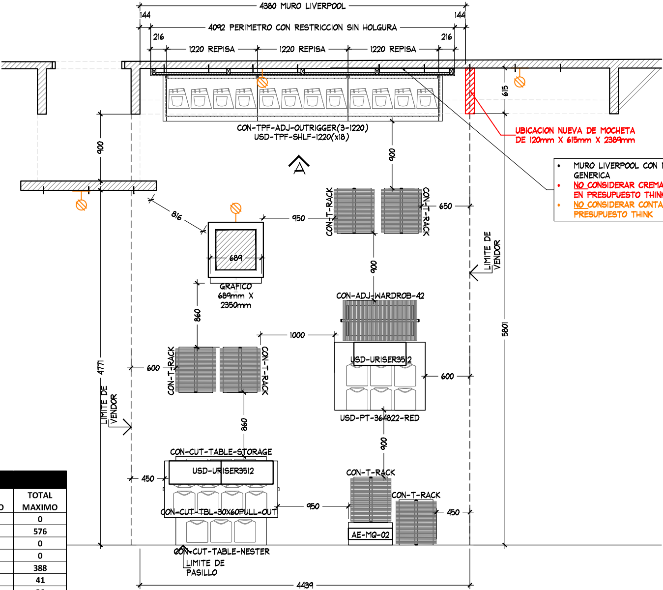
PLANTA ARQUITECTONICA ESC. 1:50
