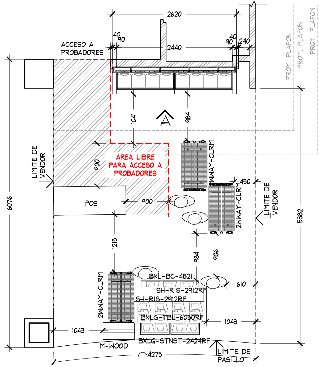
PLANTA ARQUITECTONICA ESC. 1:50
