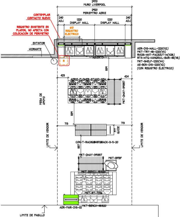
PLANTA ARQUITECTONICA ESC. 1:50
