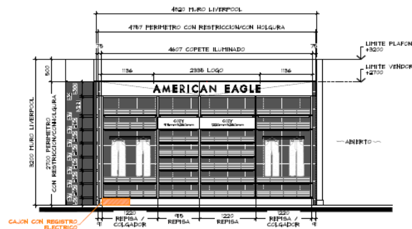
ALZADO B ESC. 1:50
