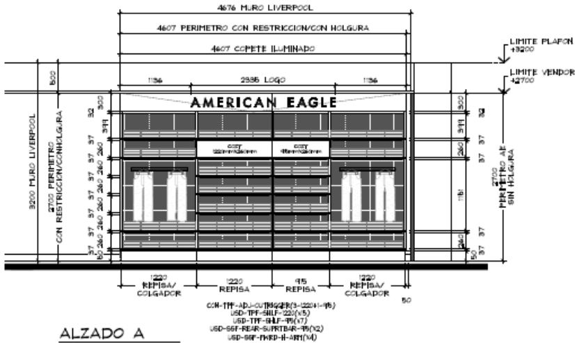
ALZADO A ESC. 1:50
