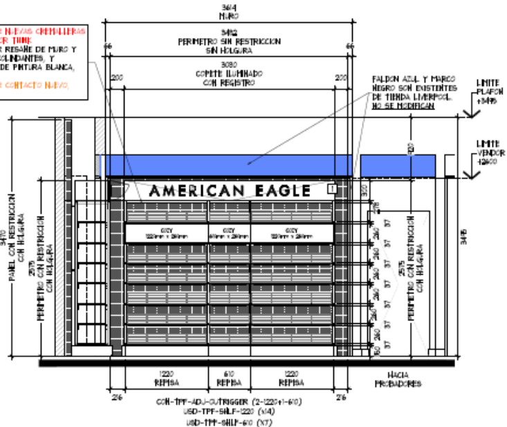
ALZADO A ESC. 1:50
