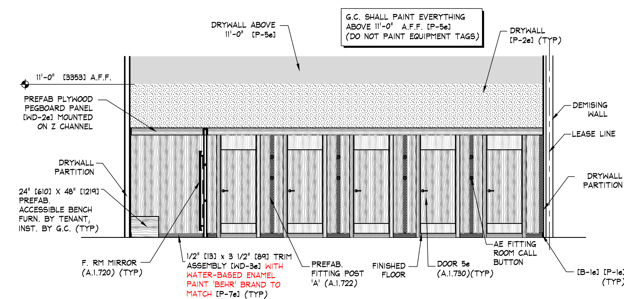
F ELEVATION A.1.601 SCALE: 1/4" = 1'-0" (1:50)
