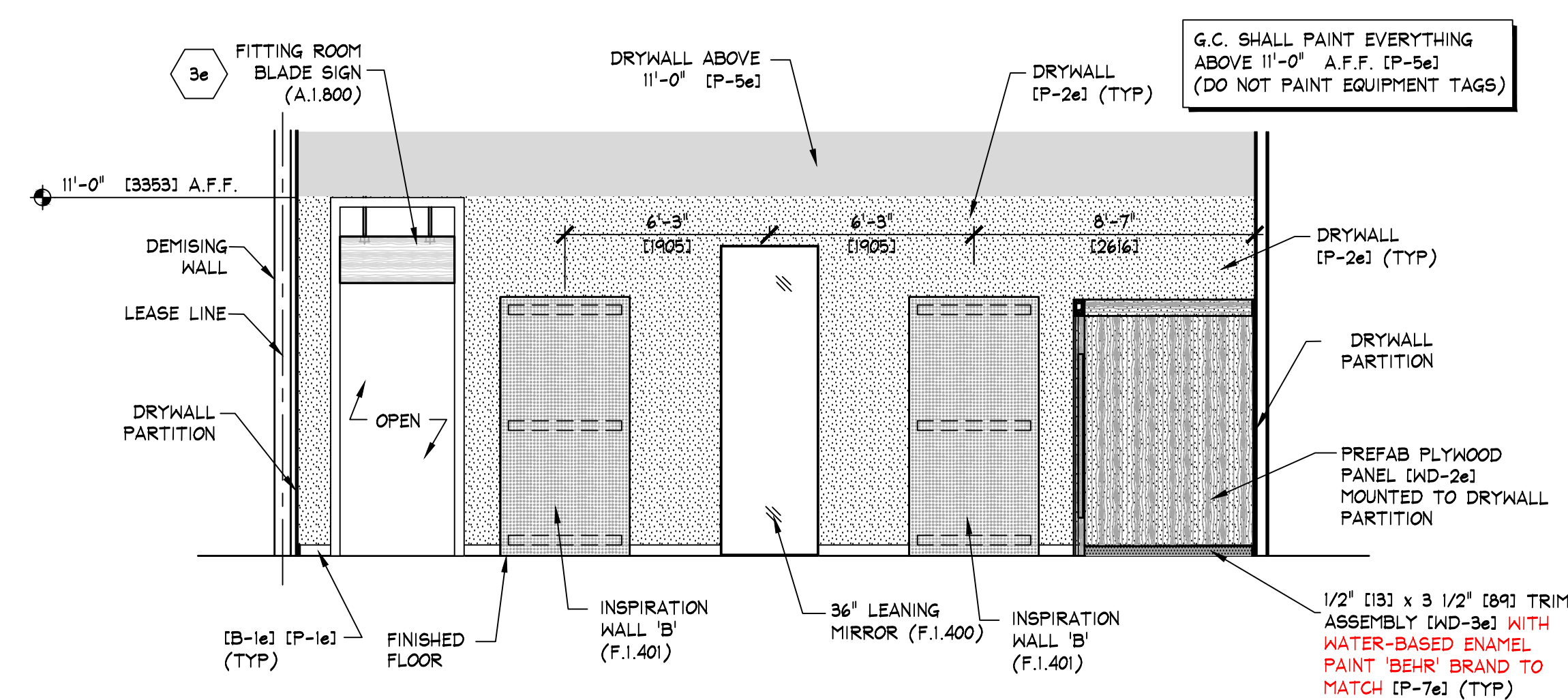
G ELEVATION A.1.601 SCALE: 1/4" = 1'-0" (1:50)
