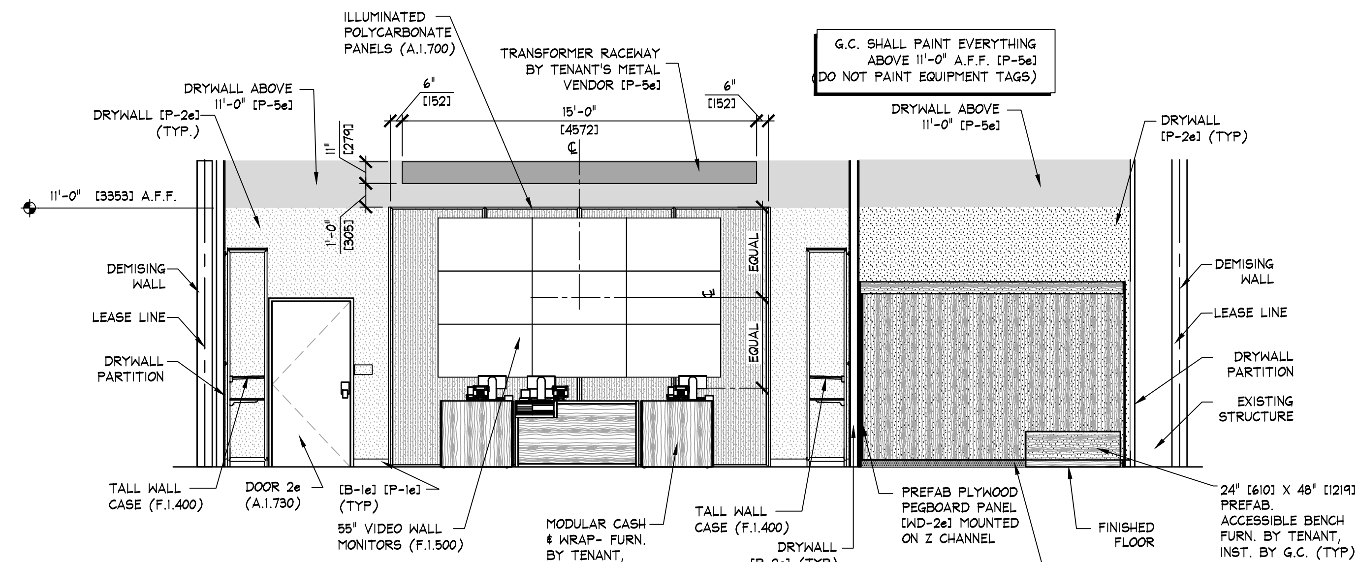
E ELEVATION A.1.601 SCALE: 1/4" = 1'-0" (1:50)
