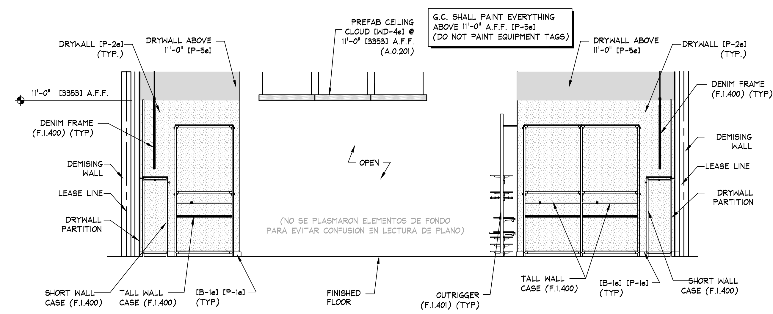
D ELEVATION A.1.601 SCALE: 1/4" = 1'-0" (1:50)
