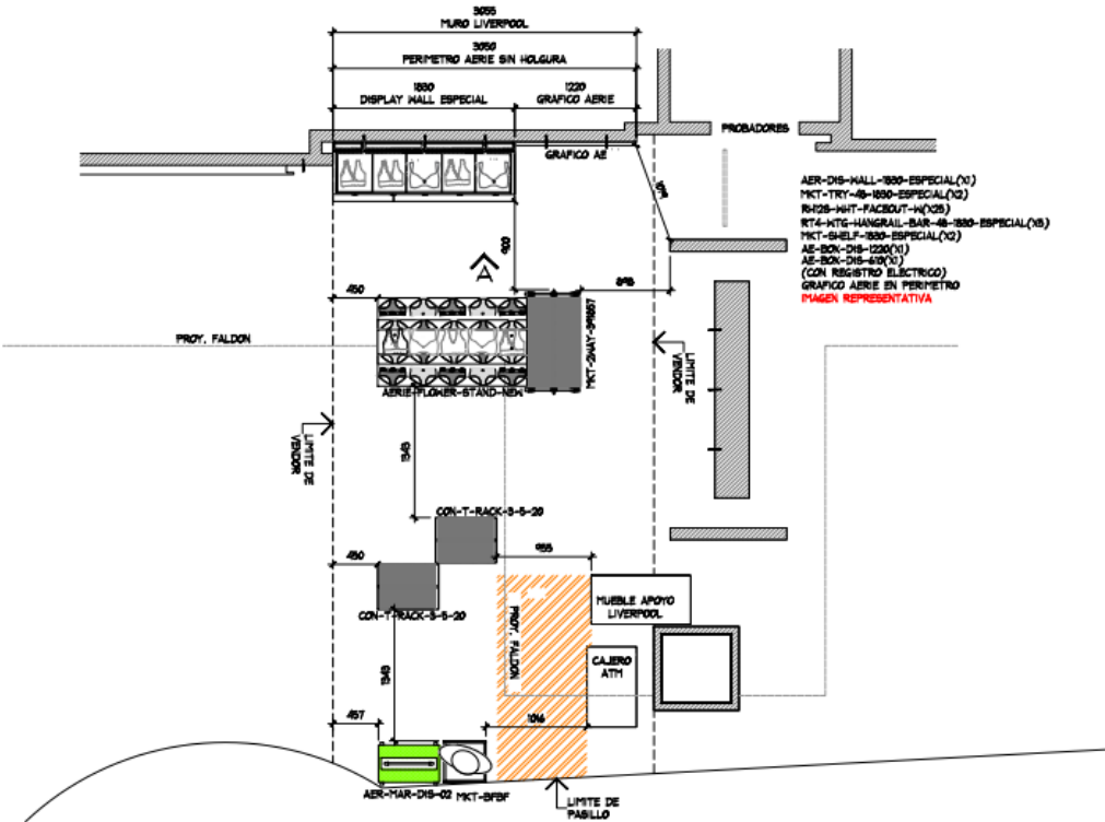
PLANTA ARQUITECTONICA ESC. 1:50
