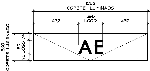
DETALLE LOGO ESC. 1:20
