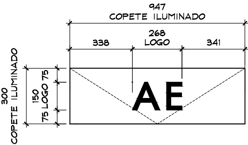
DETALLE LOGO ESC. 1:20
