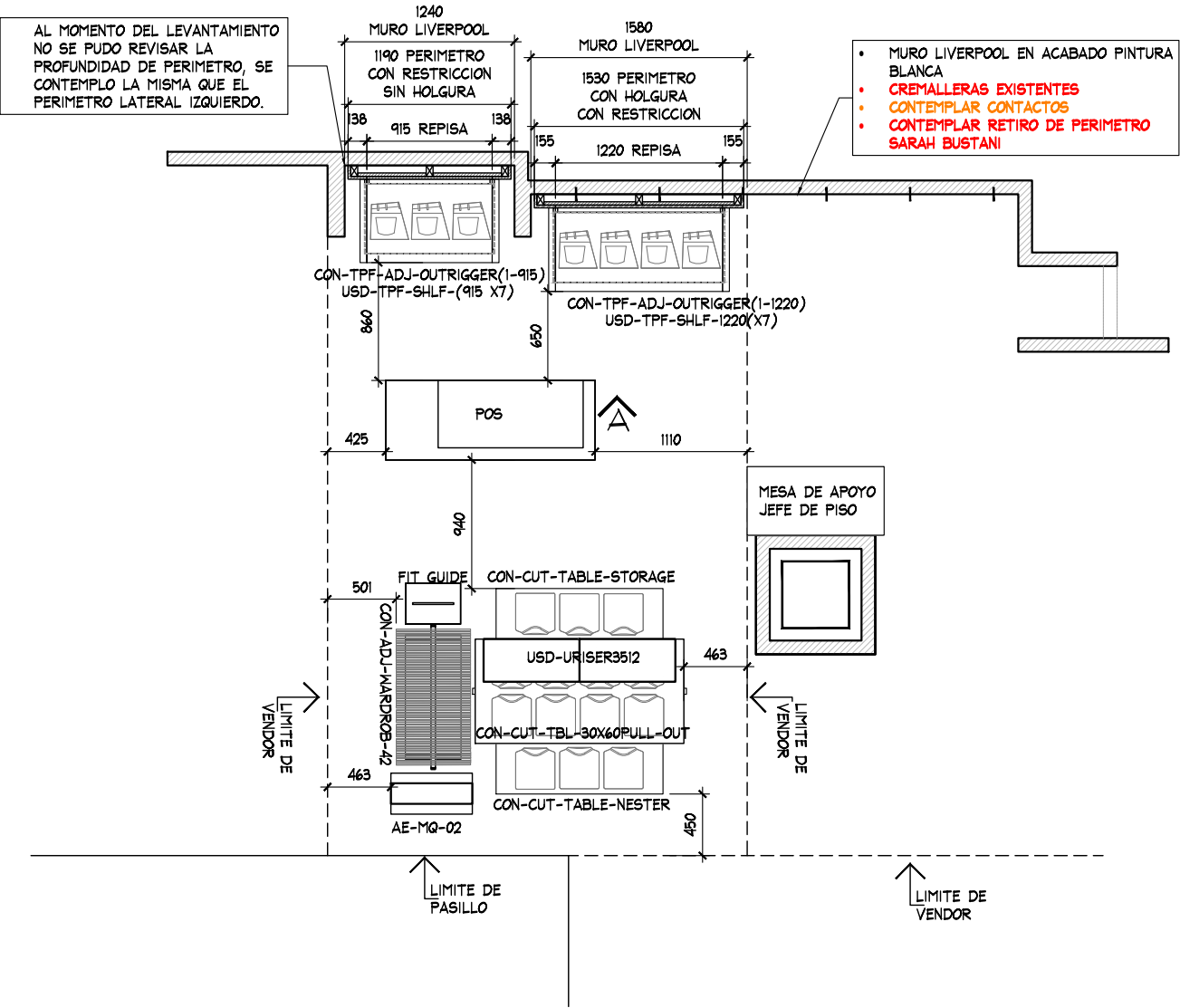
PLANTA DE ARQUITECTONICA ESC. 1:50
