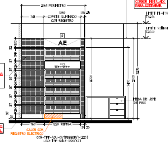
ALZADO ESC. 1:50
