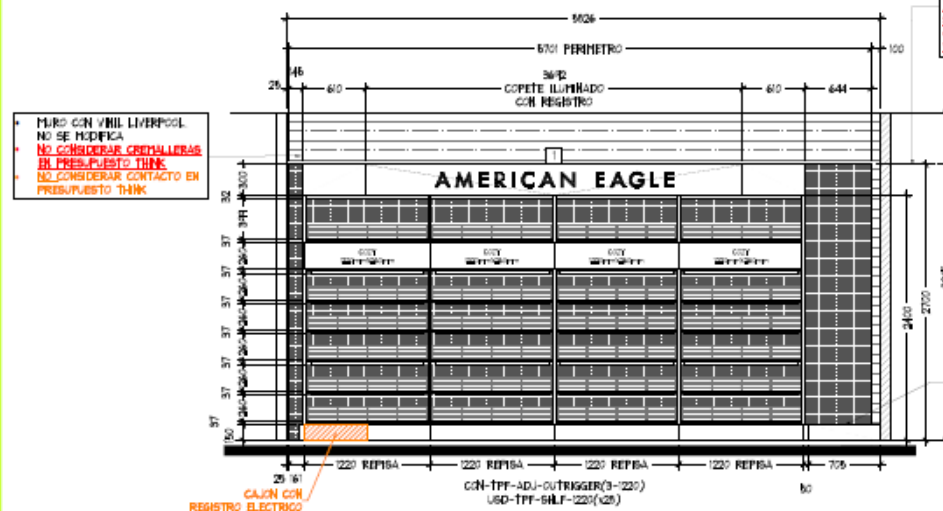
ALZADO A ESC. 1:50
