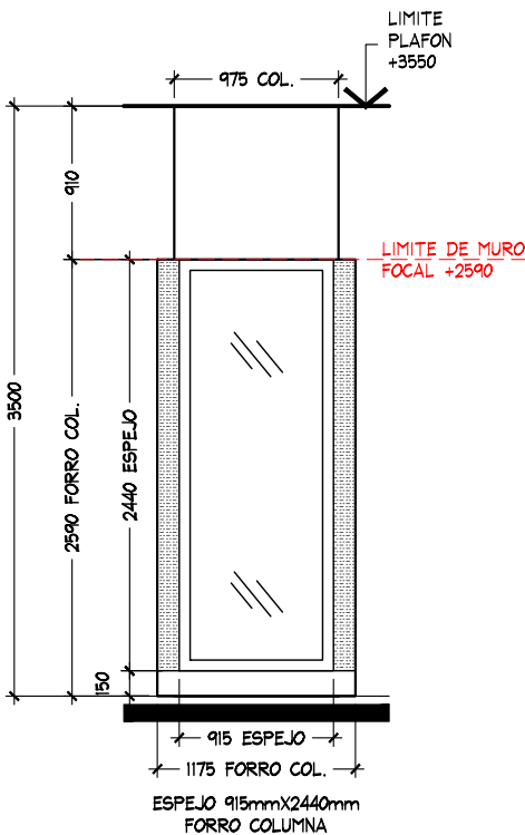
ALZADO E ESC. 1:50
