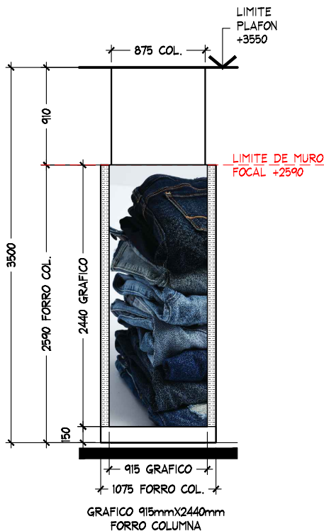
ALZADO F ESC. 1:50
