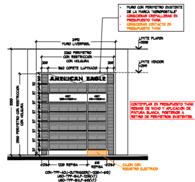
ALZADO B ESC. 1:50
