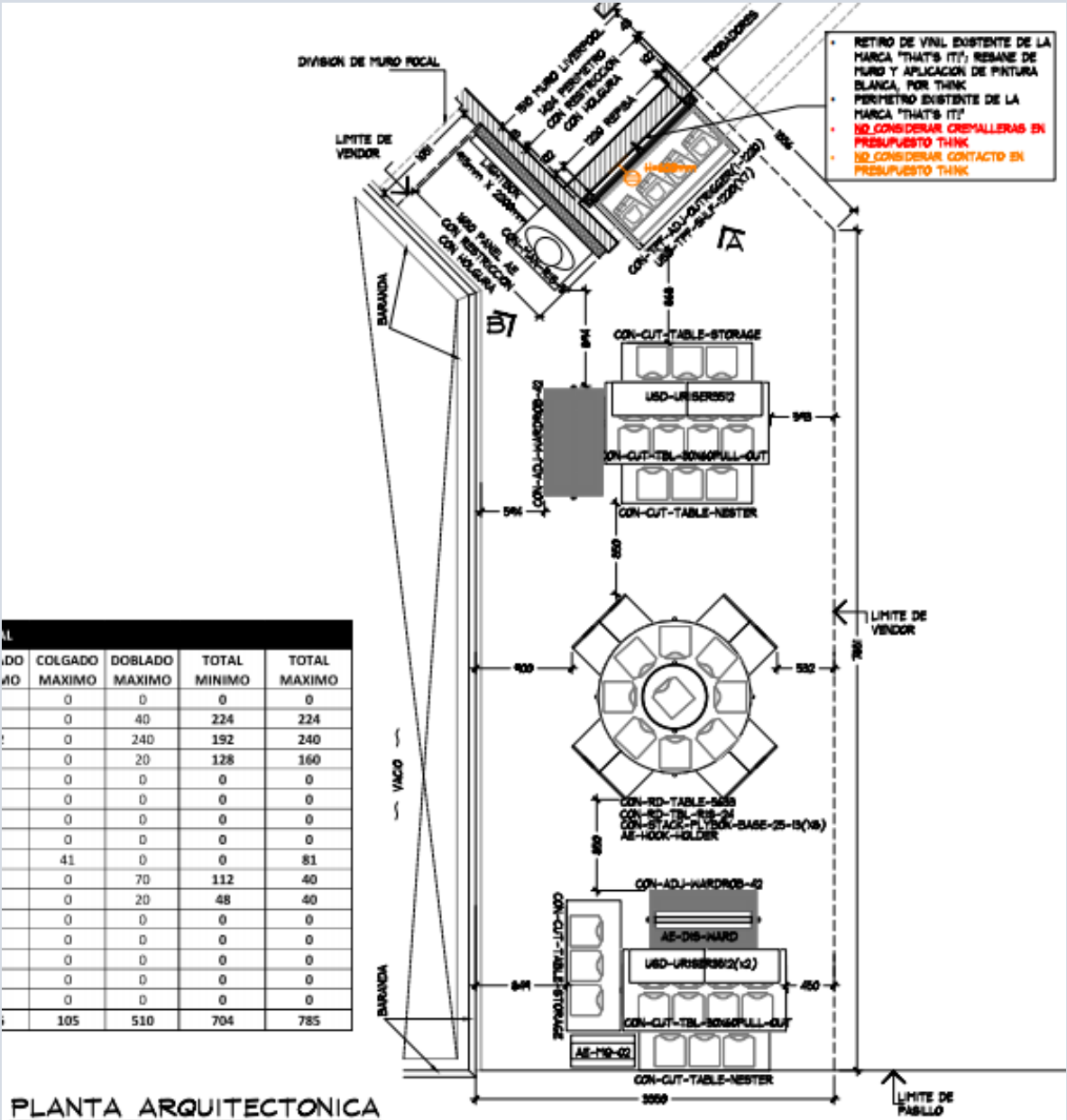
PLANTA ARQUITECTONICA
