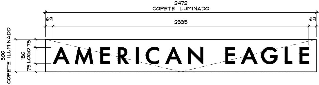
DETALLE DE LETRERO ESC. 1:20
