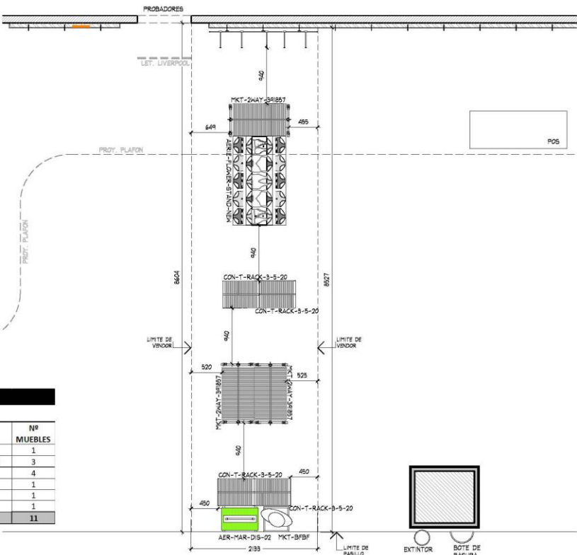
PLANTA ARQUITETONICA ESC. 1:50
