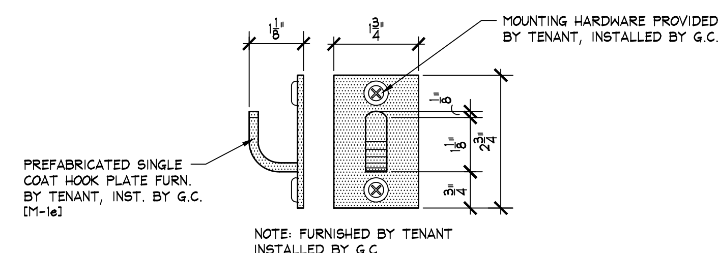
PREFAB COAT HOOK DETAIL G.1.720 SCALE: 6" = 1' - 0" [1:2]
