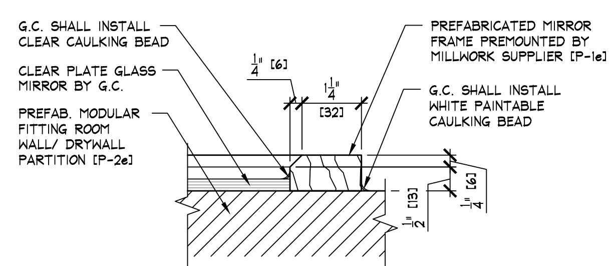
MIRROR TRIM DETAIL H.1.720 SCALE: 6" = 1'-0" [1:2]
