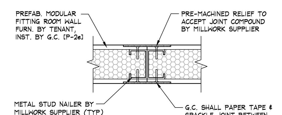
MODULAR WALL JOINT DETAIL N.1.720 SCALE: 3" = 1'-0" [1:4]
