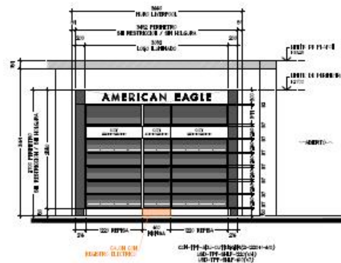
ALZADO B ESC. 150
