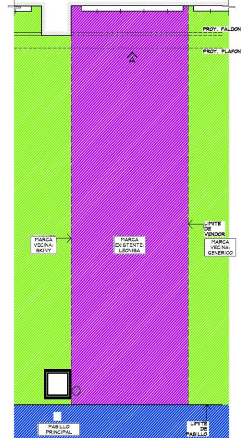
PLANTA GENERAL ESC. 1:50
