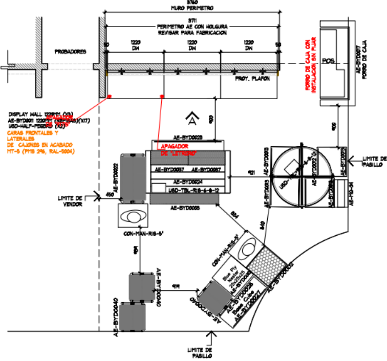
PLANTA DE MOBILIARIO ESC. 1:50
