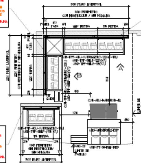
PLANTA ARQUITECTONICA ESC. 1:50
