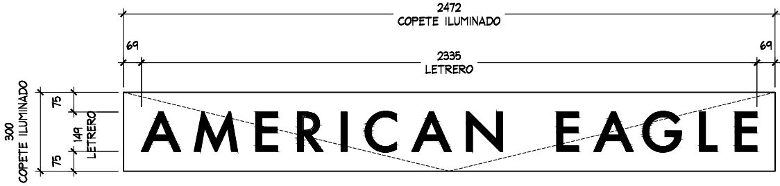
DETALLE LOGO ESC. 1:20
