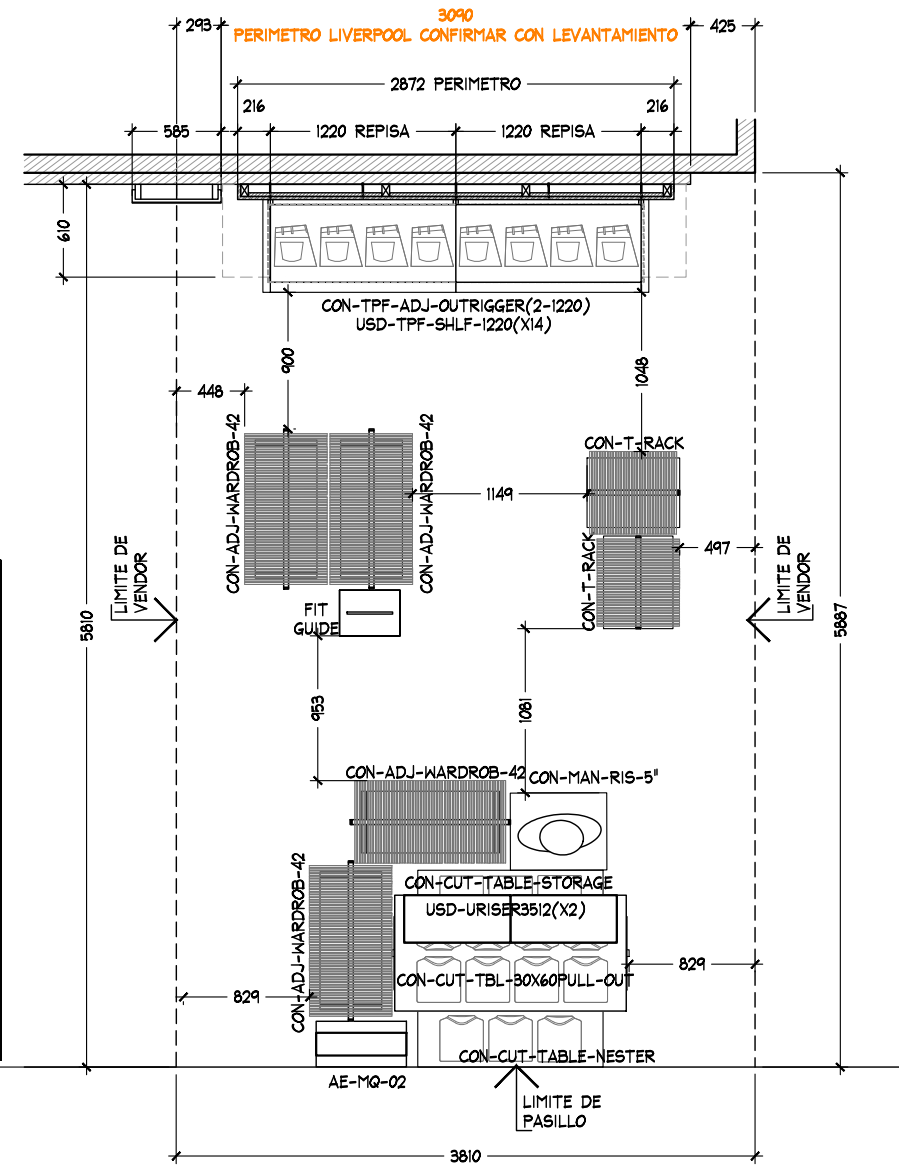
PLANTA ARQUITECTONICA ESC. 1:50
