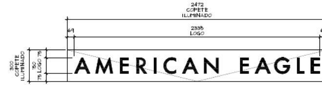
DETALLE LOGO ESC. 1:20
