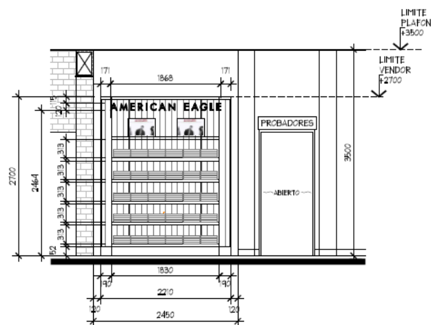
ALZADO A ESC. 1:50
