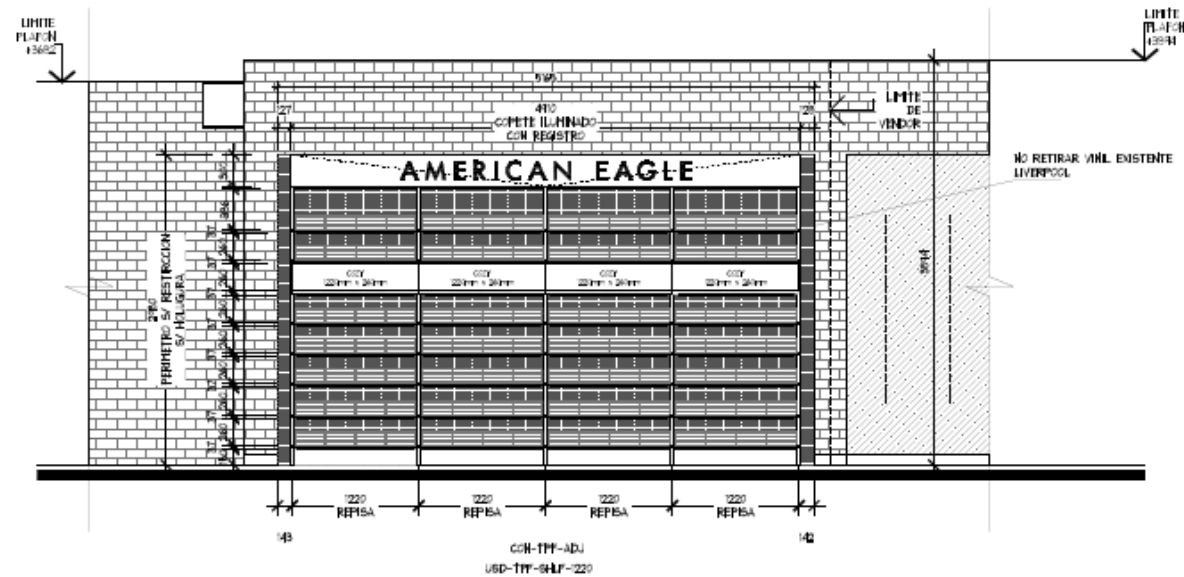
ALZADO A ESC. 1:50
