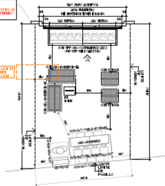
PLANTA ARQUITECTONICA ESC. 1:50
