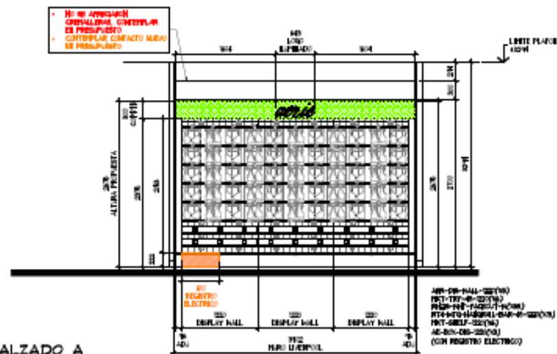
ALZADO A ESC. 1:50
