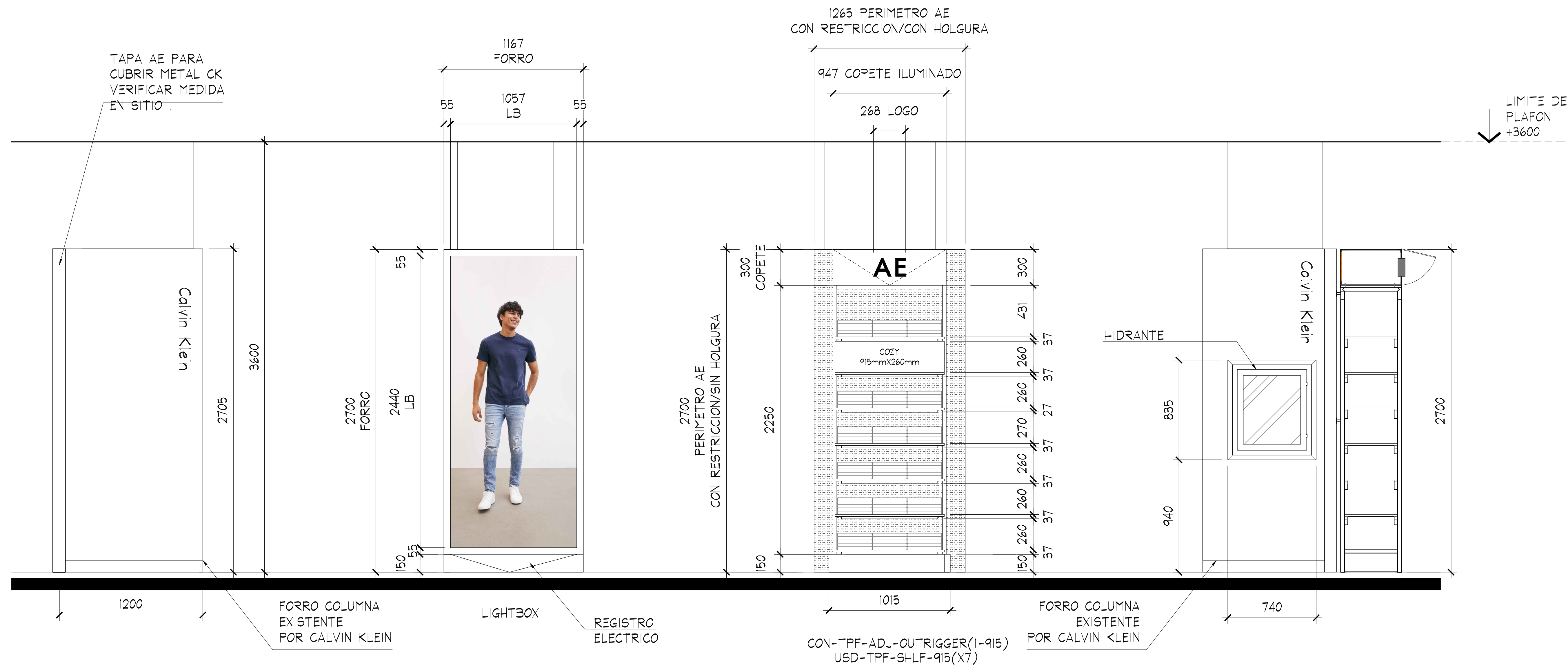
ALZADO B ESC. 1:50
