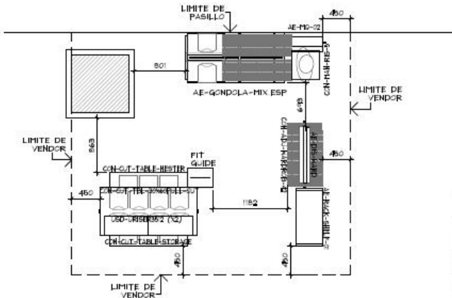
PLANTA ARQUITECTONICA ESC. 1:50
