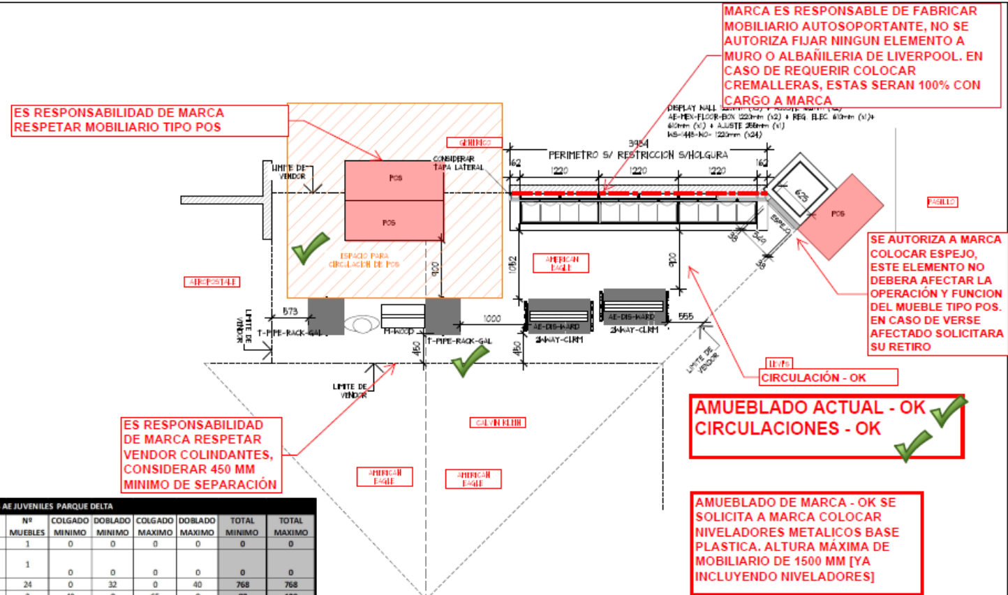
PLANTA DE MOBILIARIO ESC. 1:50
