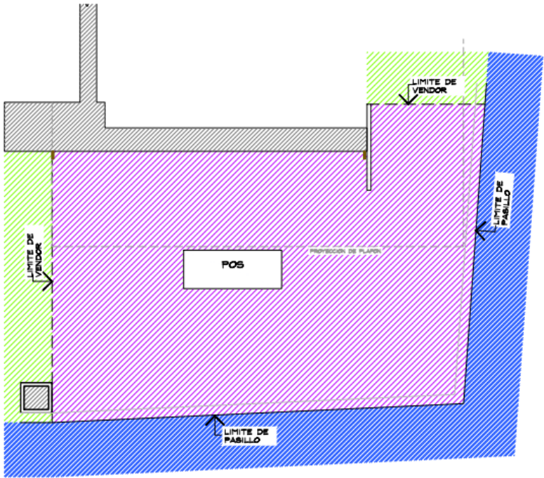
PLANTA GENERAL ESC. 1:50
