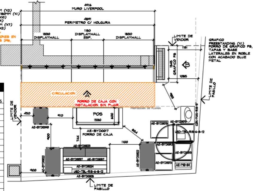
PLANTA MOBILIARIO ESC. 1:50
